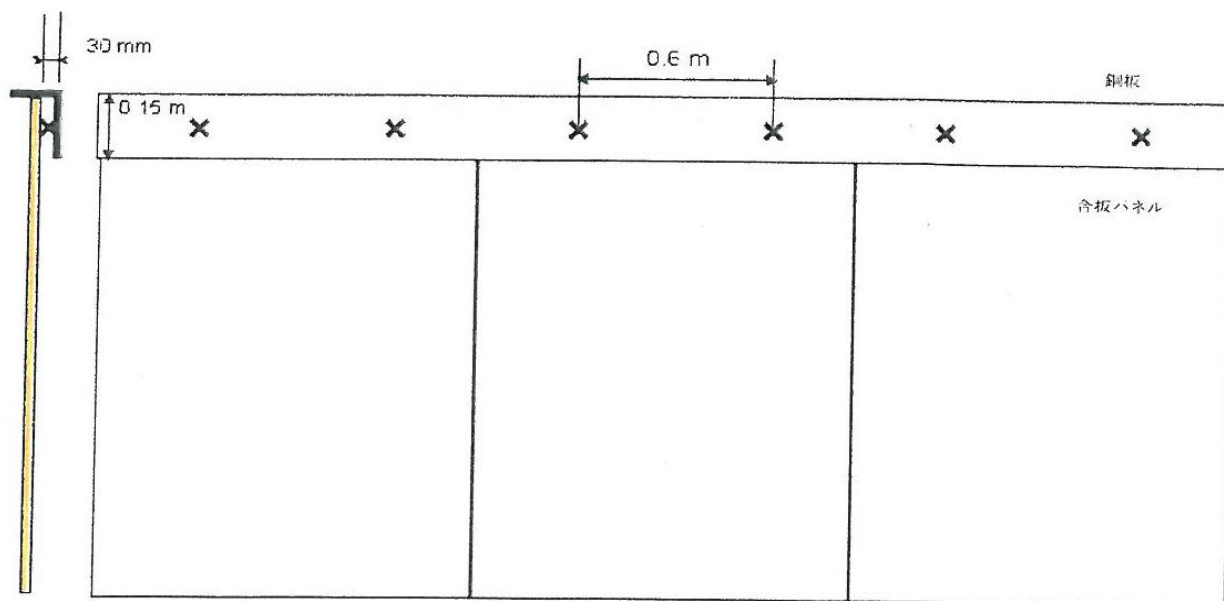
図 3.5.2 ターゲットの点火を判断するための、合板のターゲットにおける熱電対の位置 4 (※4 (約 1mm)の薄い鋼板を、図で示すように合板パネルの上端で曲げる。パネルが炭化しただけの場合には、覆いがない表面の黒く焦げた部分と金属板の下で焦げていない部分の間がくっきりとした境界として見る事ができる。火災が点火した場合には、炭化は、鋼板の下にも見られ、金属板の下のガス温度が大きく上昇していたことによって確認される。)
