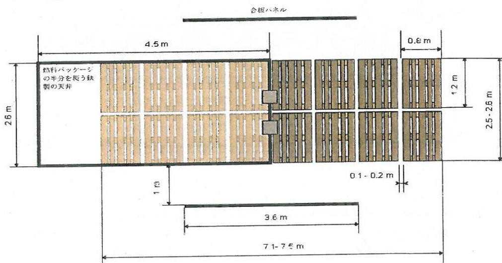
図 3.3.2.3 模擬のトラックにおける貨物燃料パッケージの上面図
