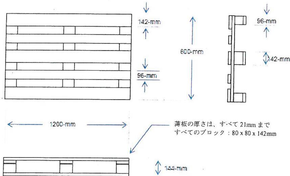
図 3.2.1 EUR の標準的な木製パレット
