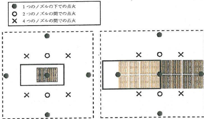
図 3.4.1 2つのシナリオにおけるノズルの位置
