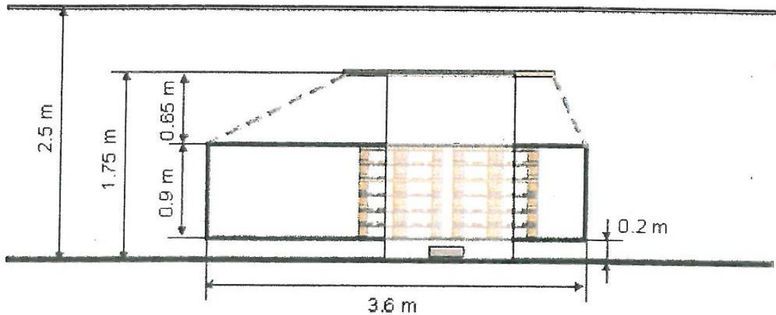
図 3.3.3.1 乗客の車両の燃料パッケージの側面図 (破線は車の形を表し、天井の板は、最も実行可能な形でその位置に固定する。)
