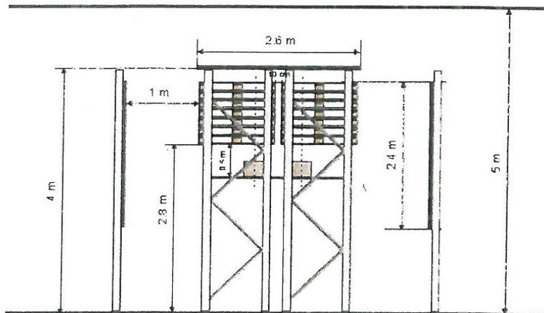
図 3.3.2.2 模擬のトラックにおける貨物燃料パッケージの端面図
