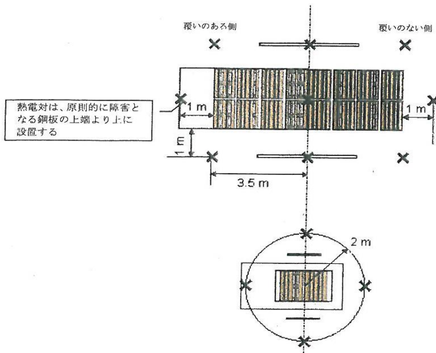
図 3.5.1 2つのシナリオにおける熱電対の位置 3
