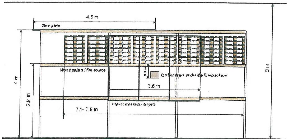
図 3.3.2.1 模擬のトラックにおける貨物燃料パッケージの側面図
