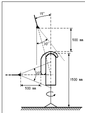
図2 不注意膨脹試験の試験配置
