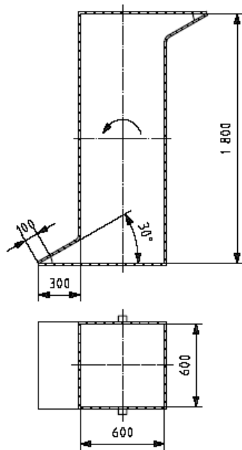
図1 回転衝撃試験装置
