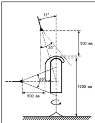
図2 不注意膨脹試験の試験配置
